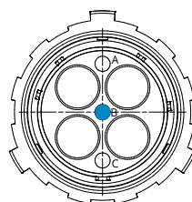
Size 40 and module number A4/I4
