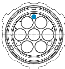
Size 48 and module n° A7/I7
